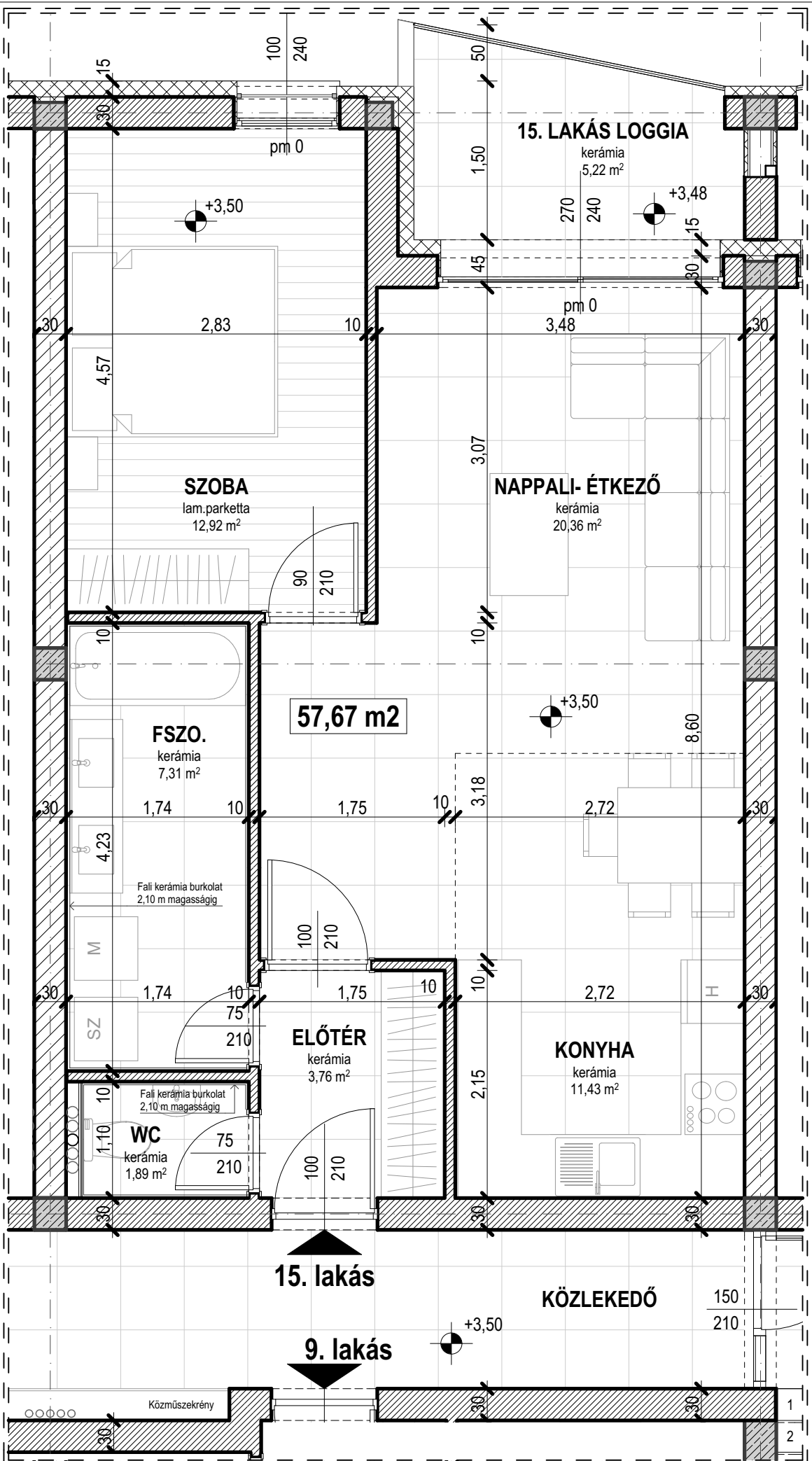
HAJDÚSZOBOSZLÓ, SZURMAI UTCA 4-6. SZ. - EMELET - 15. LAKÁS - 57,67 m²
